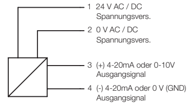
Schema/Klemmenbelegung GB 604 MF0,75
